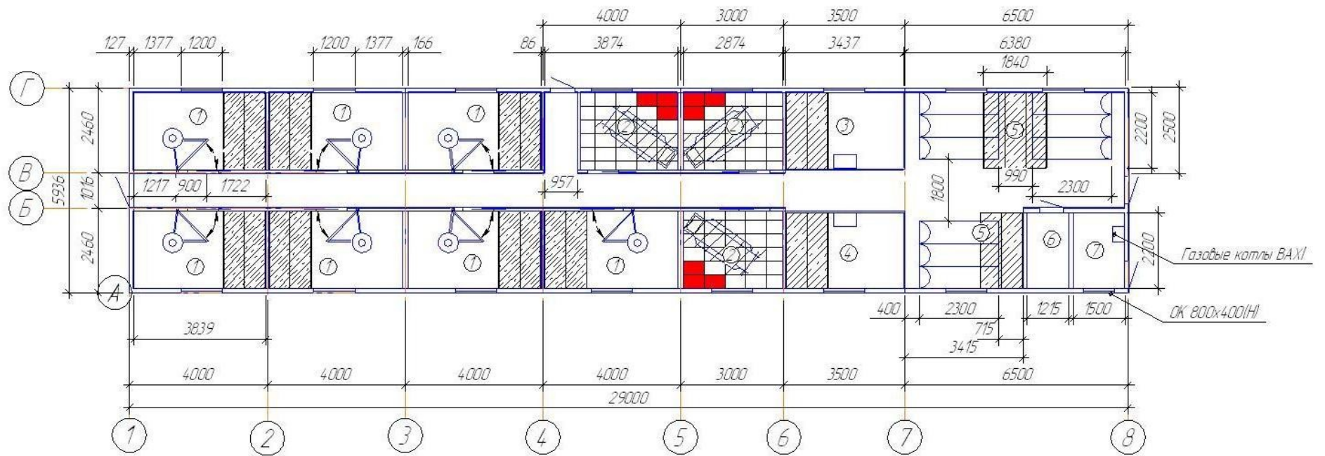
Рисунок 1 План микрофермы по выращиванию свиней
